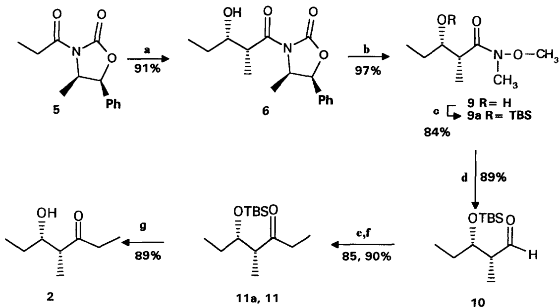
Scheme 2. (a) \text{Bu}_2\text{BOTf} , \text{Et}_3\text{N} , \text{CH}_2\text{Cl}_2 , -78^\circ\text{C} ; \text{EtCHO} ; (b) \text{AlMe}_3 , \text{MeONHMe}\cdot\text{HCl} , \text{CH}_2\text{Cl}_2 , -10^\circ\text{C} ; (c) \text{TBDMSCl} , imidazole, DMF, 25^\circ\text{C} ; (d) \text{DIBAL-H} , \text{CH}_2\text{Cl}_2 , -78^\circ\text{C} ; (e) \text{EtMgBr} , \text{Et}_2\text{O} , 0^\circ\text{C} ; (f) \text{PCC} , \text{NaOAc} , \text{CH}_2\text{Cl}_2 ; (g) tetrabutylammonium fluoride, THF, 25^\circ\text{C} .
