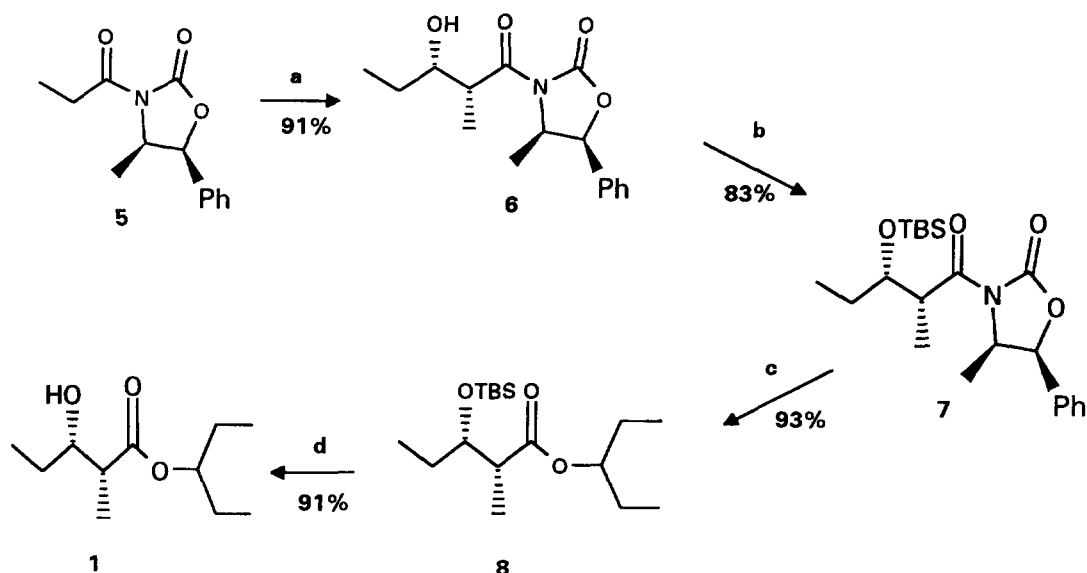
Scheme 1. (a) \text{Bu}_2\text{BOTf} , \text{Et}_3\text{N} , \text{CH}_2\text{Cl}_2 , -78^\circ\text{C} , \text{EtCHO} ; (b) \text{TBDMSCl} , imidazol, DMF, 25^\circ\text{C} ; (c) \text{LiOCH}(\text{Et})_2 , THF, 0^\circ\text{C} ; (d) tetrabutylammonium fluoride, THF, 25^\circ\text{C} .
